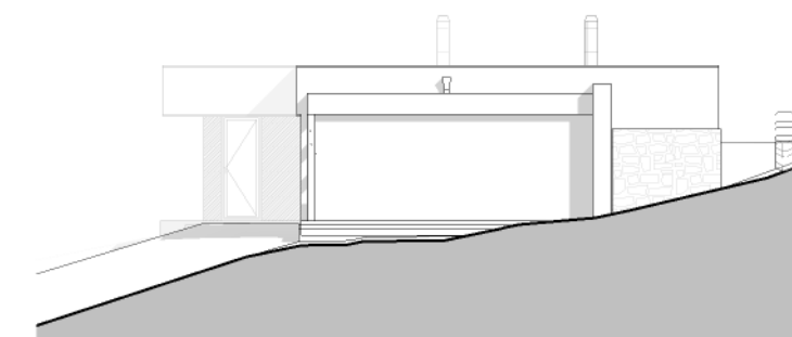
6 1:200 POHL'AD č.3
