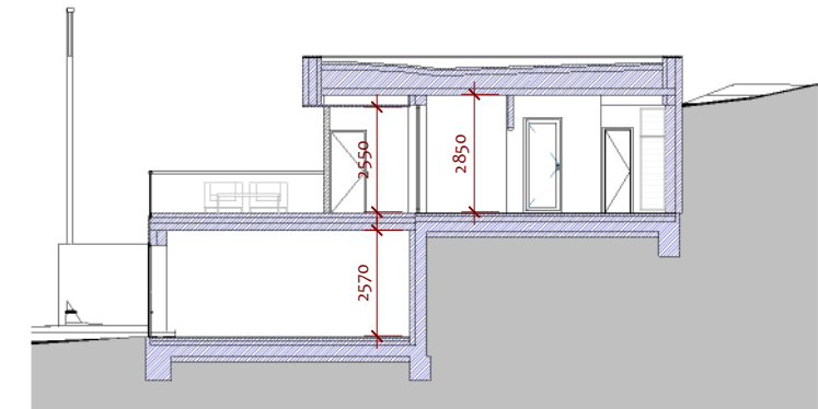
4 1:200 PRIEČNY REZ
