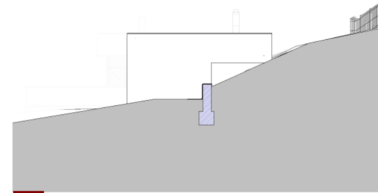
7 1:200 POHLAD č.3
