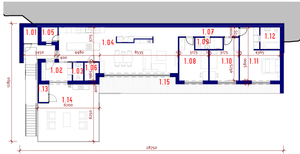
2 1:200 PÓDORYS 1.NP
